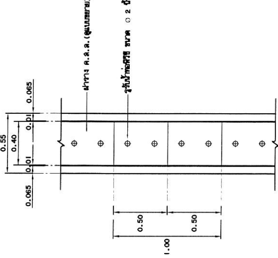
ขยายฝักรางระบายน้ำ ค.ส.ล.ใหม่
